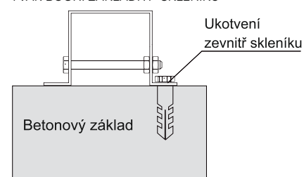
TVAR BOČNÍ ZÁKLADNY SKLENÍKU
