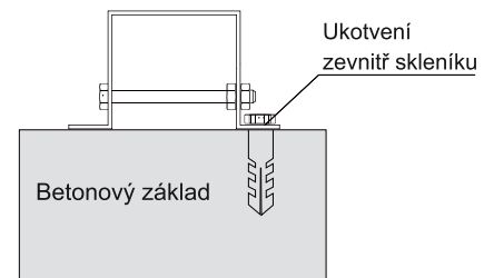
TVAR BOČNÍ ZÁKLADNY SKLENÍKU
