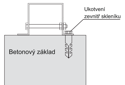
TVAR BOČNÍ ZÁKLADNY SKLENÍKU
