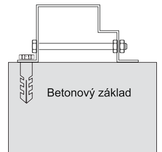
TVAR ČELNÍ ZÁKLADNY PRO TYP J
