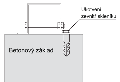
TVAR BOČNÍ ZÁKLADNY SKLENÍKU
