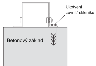
TVAR BOČNÍ ZÁKLADNY SKLENÍKU
