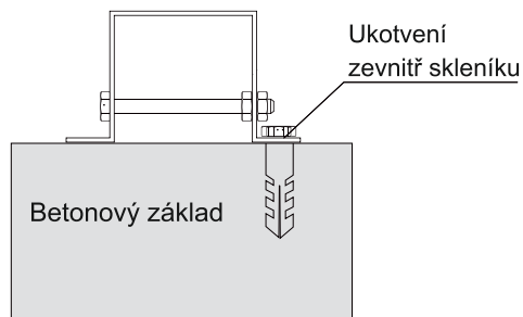
TVAR BOČNÍ ZÁKLADNY SKLENÍKU VARIANT
