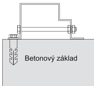
TVAR ČELNÍ ZÁKLADNY PRO TYP K
