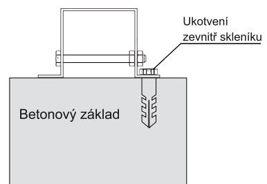
TVAR BOČNÍ ZÁKLADNY SKLENÍKU VARIANT
