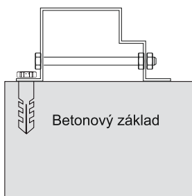
TVAR ČELNÍ ZÁKLADNY PRO TYP J
