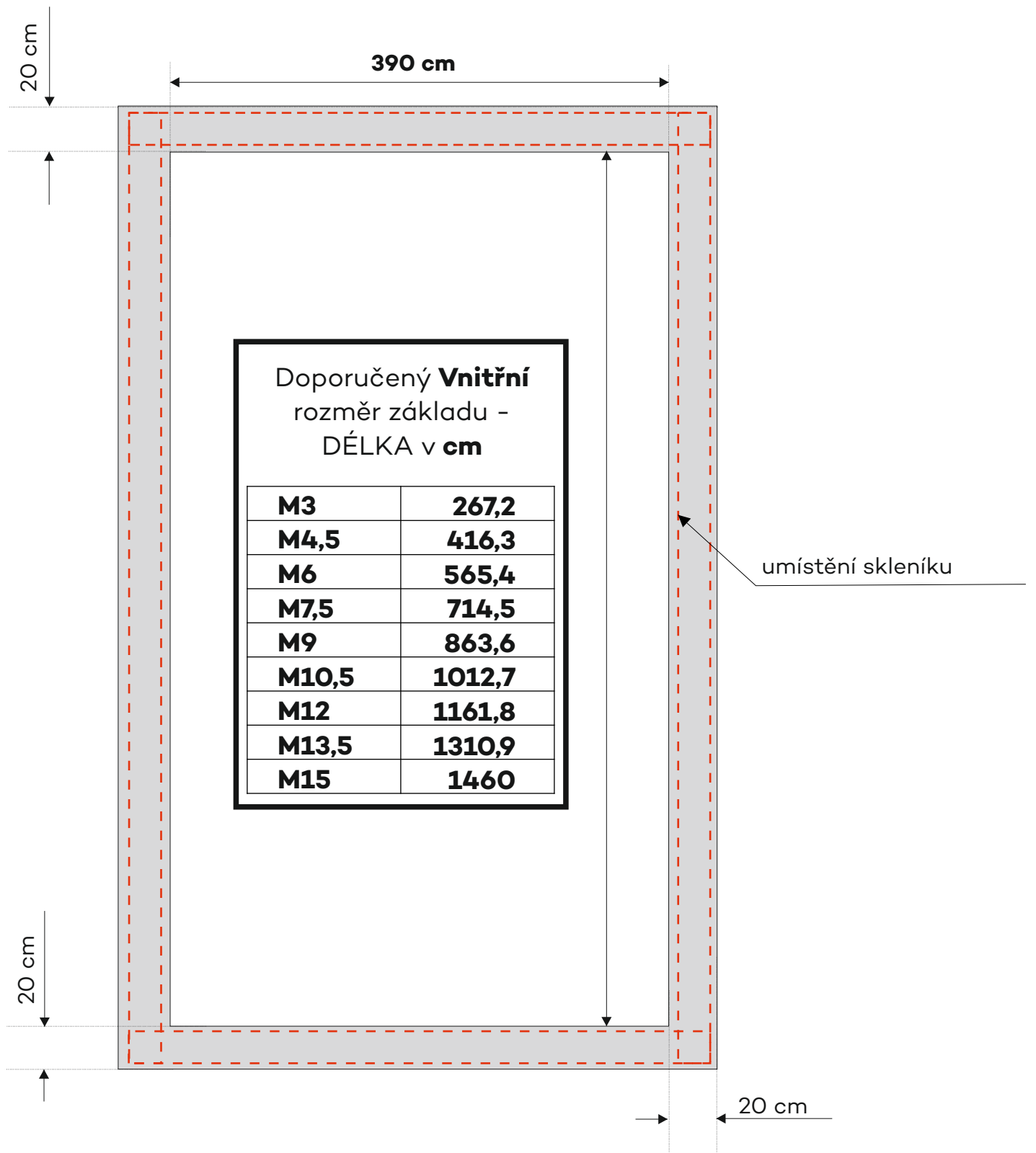
BOČNÍ A ČELNÍ ZÁKLADNA PRO TYP L
