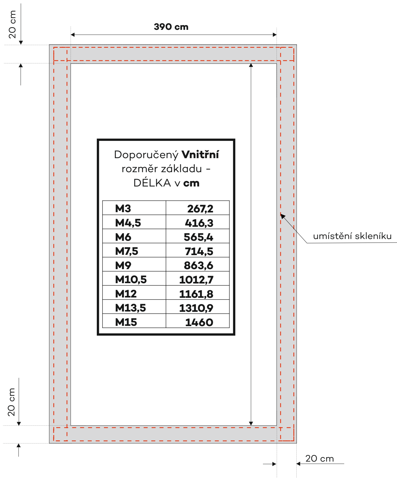
BOČNÍ A ČELNÍ ZÁKLADNA PRO TYP L
