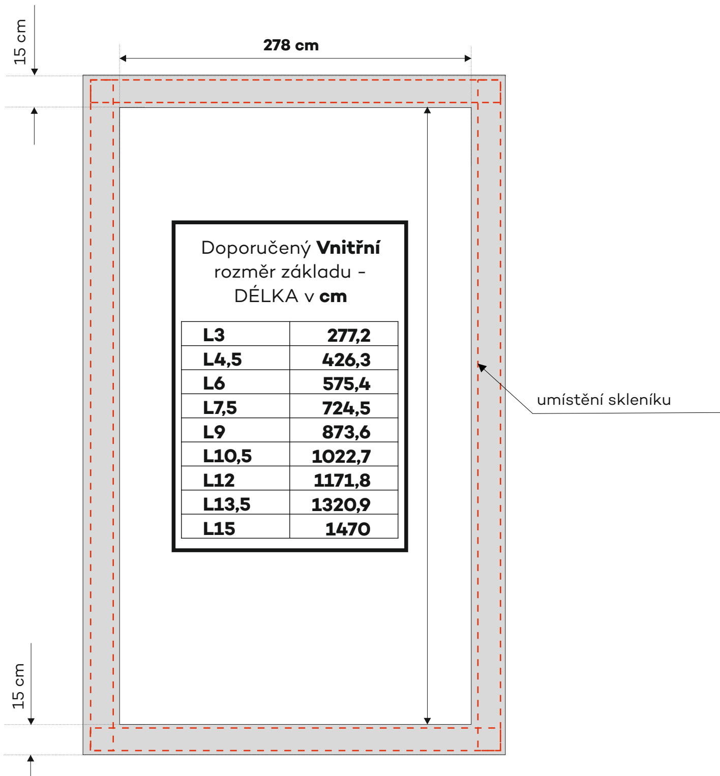
BOČNÍ A ČELNÍ ZÁKLADNA PRO TYP L
