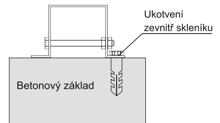
TVAR BOČNÍ ZÁKLADNY SKLENÍKU VARIANT
