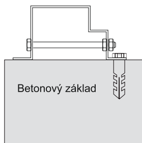
TVAR ČELNÍ ZÁKLADNY PRO TYP J
