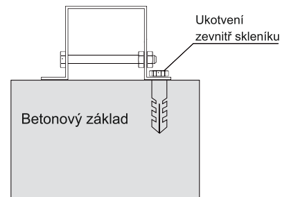
TVAR BOČNÍ ZÁKLADNY SKLENÍKU VARIANT
