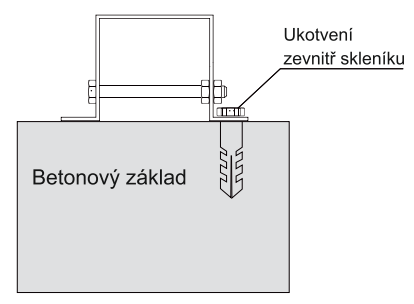
TVAR BOČNÍ ZÁKLADNY SKLENÍKU VARIANT
