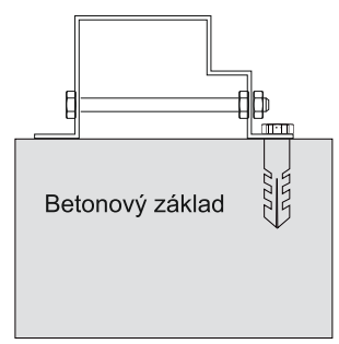
TVAR ČELNÍ ZÁKLADNY PRO TYP J
